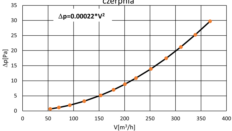
Charakterystyka hydrauliczna nawiewnik K5 czerpnia
