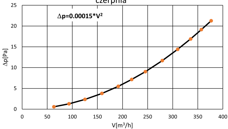
Charakterystyka hydrauliczna nawiewnik K4 czerpnia
